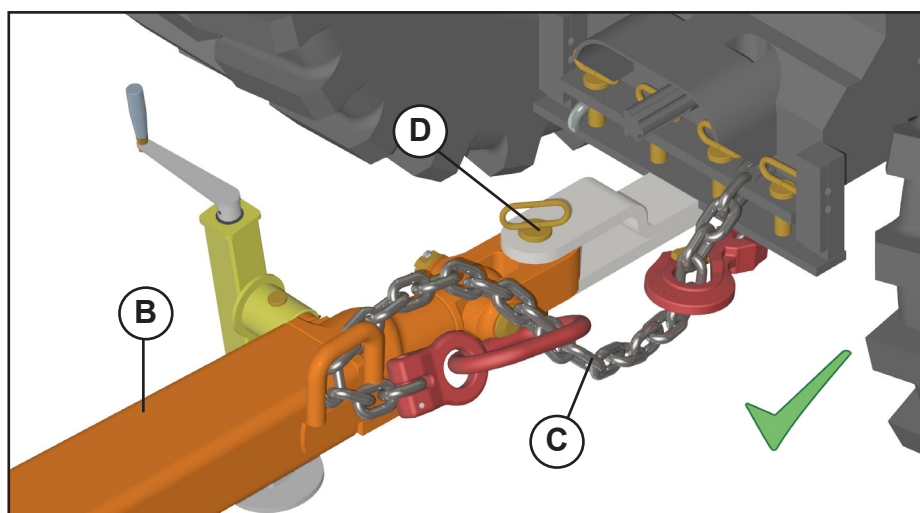
Correto
